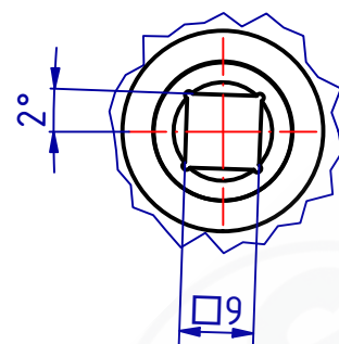
A ( 1 : 1 )
