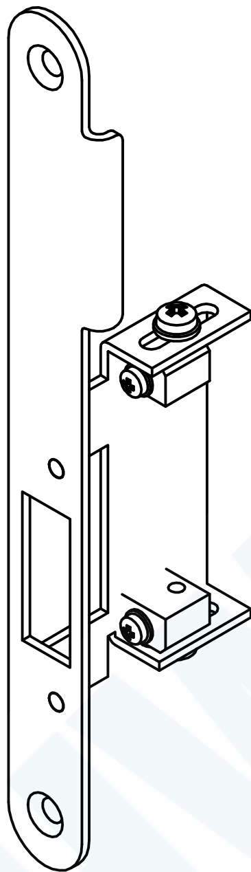
124887 Riegelschließblech GSV-Nr. 5626 R S015 links Edelstahl rostfrei gebürstet 2J 2 mm dick lasergeschnitten passend zu Schnappschalter EDV-Nr.124822 nach Zeichnung vom 3.5.22 Index - 124887 Dead bolt strike plate GSV-No. 5626 S015 left hand stainless steel brushed 2J 2 mm thick laser cut suiting to snap action switch EDP-No. 124822 in accordance with drawing 3.5.22 Index -
