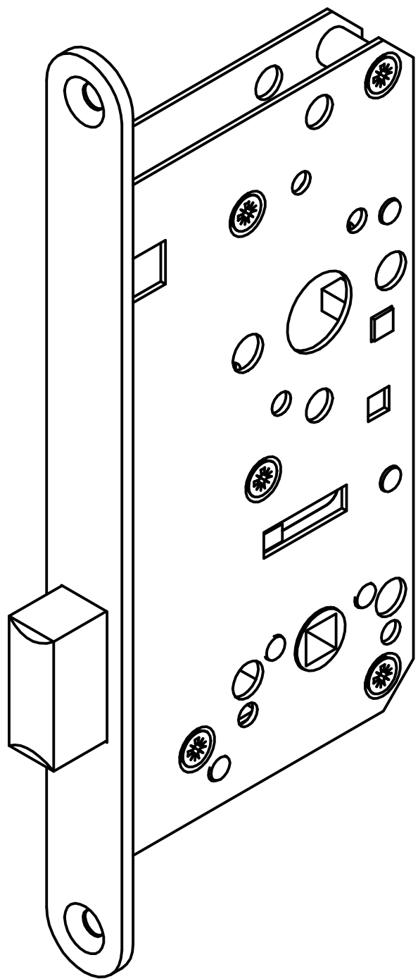
124820 Einsteck-WC-Riegelschloss Dorn 55mm GSV-Nr. 3801 WCR S008 ohne Schließblech Nußloch nicht gezogen Schlüsselbahn nicht gedrückt 8mm WC-Nuss Stulp 20 x 210 x 3 mm Edelstahl rostfrei gebürstet 2J Zeichnung vom 03.5.22 Index b vom 22.06.22 Betätigungsmoment WC-Nuss: <0.55Nm (20N auf einer Länge von 27,5mm) Betätigungsmoment in nicht eingebauten Zustand 124820 Mortise WC-latchlock backset 55mm GSV-No. 3801 WCR S008 right hand without strike plate nuthole not drawn key line not pressed 8 mm WC-hub front plate 20x210x3 mm stainless steel brushed 2J drawing 03.5.22 Index b dating 22.06.22 Operating torque WC-hub: <0.55Nm (20N on leverage length 27,5mm) all operation torques for unmounted lock
