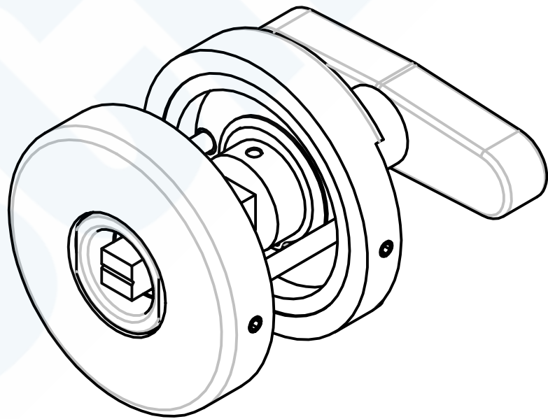
124863 WC-Roses Set WCP GSV-Nr. 1400 WCP S004 A Edelstahl rostfrei gebürstet 2J durchgehende Hülsenschrauben taktile rot/grün Anzeige Innenseite Blindabdeckung nach Zeichnung vom 3.5.22 Index -
