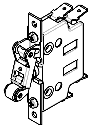
124822 Schnappschalter Wechsler mit Doppelunterbrechung und Zwangsöffnung 124822 snap-action switch changeover switches with double break contacts and positive opening operation
