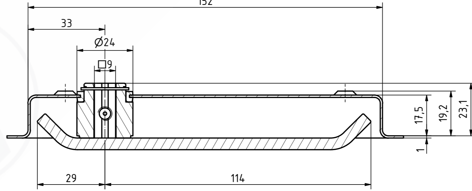
A-A ( 1 : 1 )
