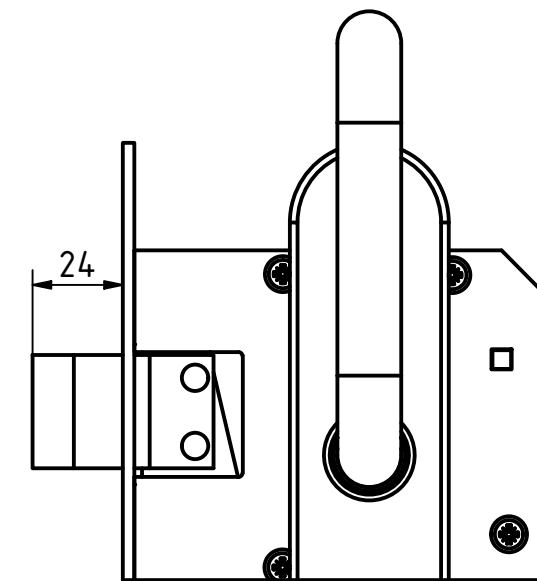
Falle ausgefahren
