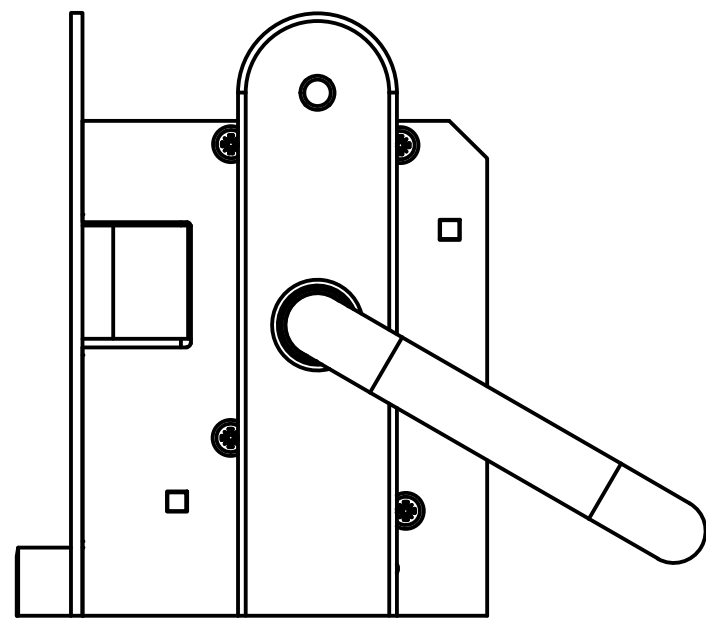
Falle eingezogen
